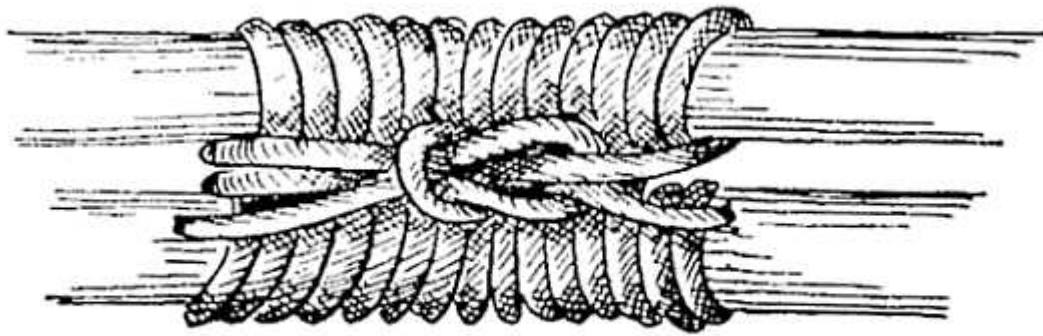
FIG. 101.—Necklace tie.
