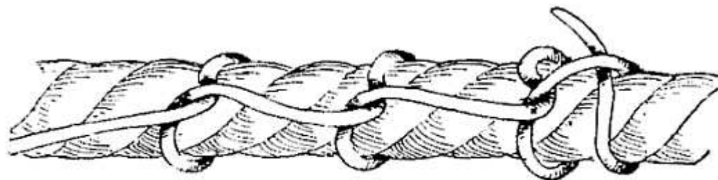
FIG. 46.—Chain hitch.
