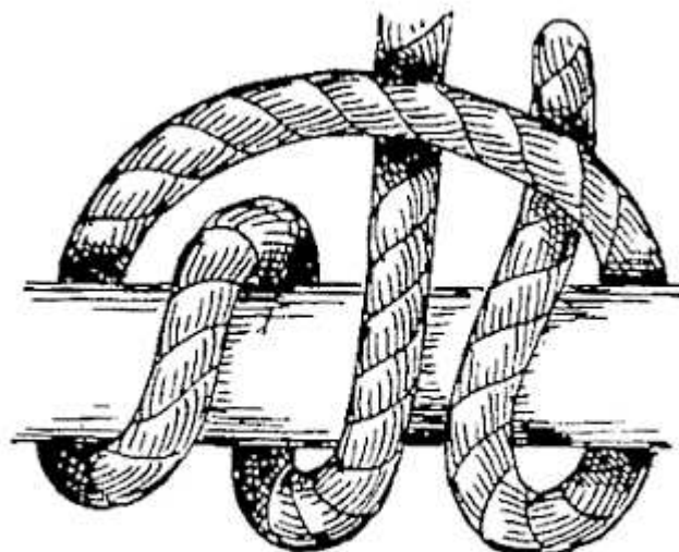
FIG. 49.—Magnus hitch.
