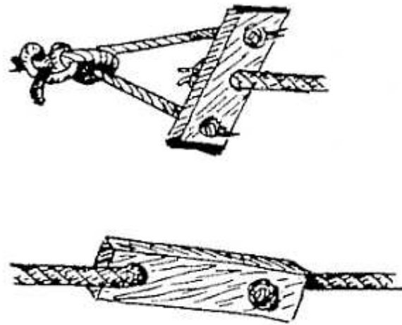
FIG. 145.—Swivels.
